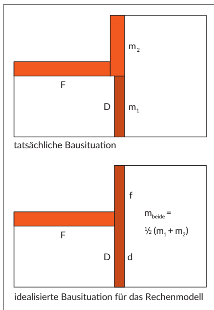
Bild 4.5: Anleitung zur Berechnung des Stoßstellendämm-Maßes bei ungleichen flächenbezogenen Massen der flankierenden Bauteile.
