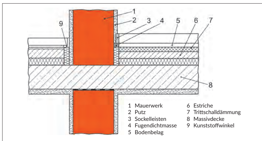
Bild 6.3: Schwimmender Estrich auf den Podesten (Schnitt A-A).
