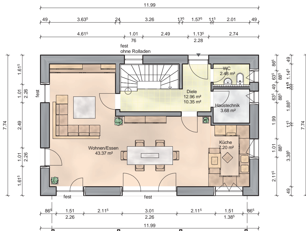
Bild 5: Grundriss des Erdgeschosses.
