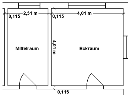
Bild 2: Den Musterrechnungen zugrunde liegende Raumanordnung
