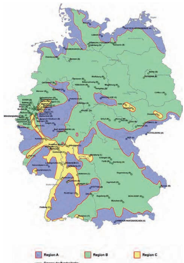
Bild 1: Sommerklimaregionen nach DIN 4108-2
