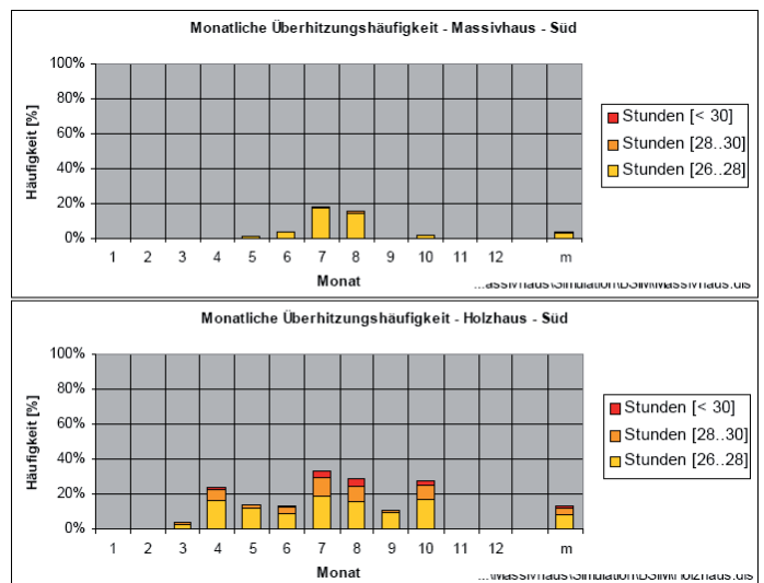
Bild 9: Häufigkeiten monatlicher Überhitzungsstunden über 26 °C für Massivhaus und Leichtbauweise nach [2].
