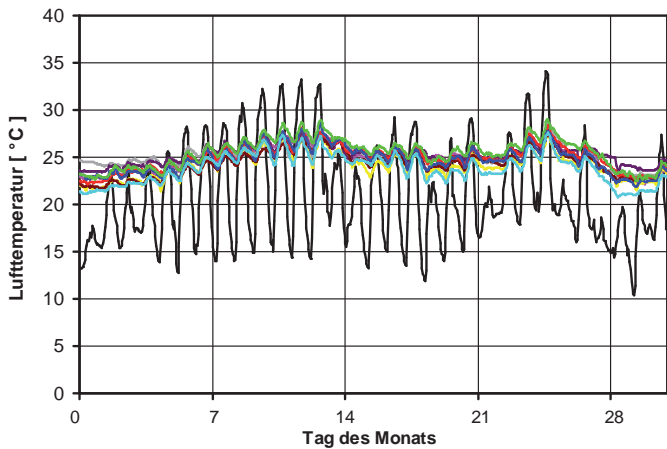
Bild 7: Tagesgang der Außenlufttemperatur (schwarz) und der mittleren Gebäudetemperaturen der 9 Niedrigenergiehäuser (farbig) im August nach [1].
