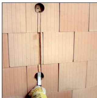
Vorgesägte Schlitzte mit Hammer und Meißel freischlagen.
