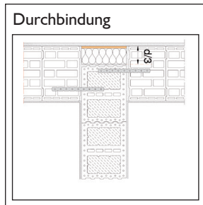
Die Durchbindung mit Dämmstoff und nur Ziegelblende an der Außenseite stellt die für den Schallschutz beste Variante dar.
