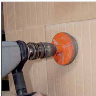
Elektrodose anzeichnen und mit handelsüblicher Bohrmaschine und Diamant-Trocken-Bohrkrone Kernbohrung vornehmen.
