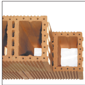
Im Mauerverband versetzt stehen die Kanäle exakt übereinander. Das ist wichtig für die geschoßhohe Betonverfüllung!
