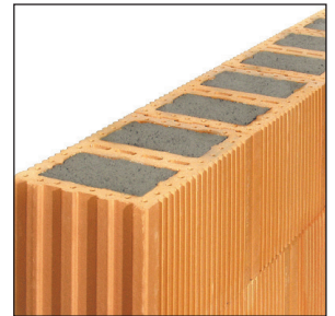
Schnelles Bauen ohne aufwendigen Materialwechsel bei Schallschutzwänden. Die fertige Planfüllziegel-Wand bringt hohe Werte im Schallschutz und in der Druckfestigkeit.
