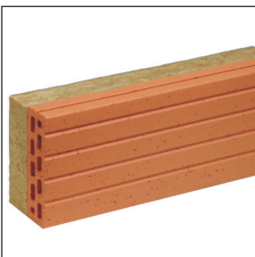
Deckenrandschale mit werksseitig aufgeklebter Isolierung, einer speziellen, hydrophobierten Mineralwolle (WLG: 035), gegen Schalungsdruck.
