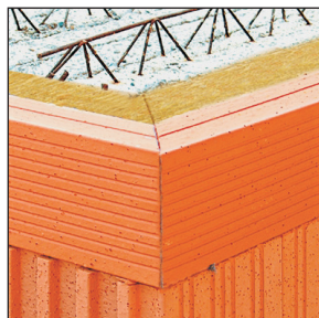
Rationelles Verlegen der Deckenrand-Systeme in einem Arbeitsschritt. Kein Zeitverlust durch Einschaltungsarbeiten.
