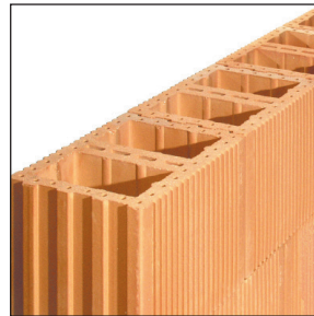
Erst die fertig gemauerte Wand wird geschoßhoch mit Beton verfüllt. Am rationellsten geht das z.B. in einem Arbeitsgang beim bzw. vor dem Betonieren der Decke.
