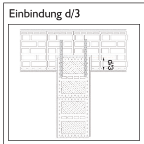
Für den geringen Anspruch an den Schallschutz (nur Mindestschallschutz nach DIN 4109-1:2018-01 gefordert) kann die Einbindung ausreichend sein. Es ist immer ein Nachweis für die individuelle Ausführungssituation erforderlich.
