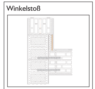
Ist die Außenwand abgewinkelt, dann ist die Durchbindung über die Außenwand hinaus mit Zusatzdämmung die für den Schallschutz beste Variante.
