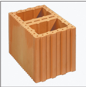
Der neue PFZ macht Anfänger überflüssig - ein Schnitt durch die Lochreihe im Mittelsteg schafft exakt 2 halbe Ziegel. Ecken, Tür- und Fensterrahmen sowie Aufzugsschächte können so noch leichter hergestellt werden als bisher.
